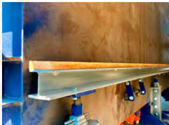
Sistema de regulación en altura y lateral
